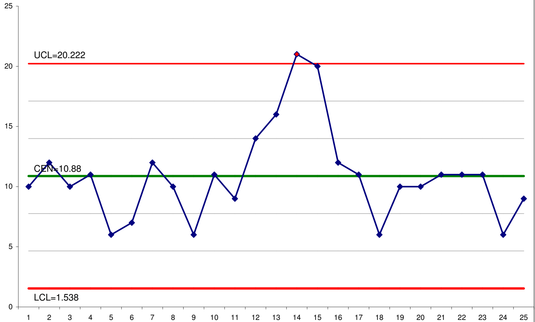
np Chart
